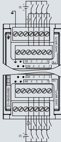
6ES7 221-1BH30-0XB0
