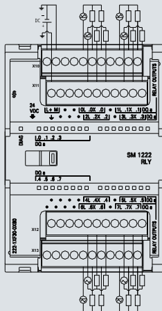
6ES7 222-1XF30-0XB0
