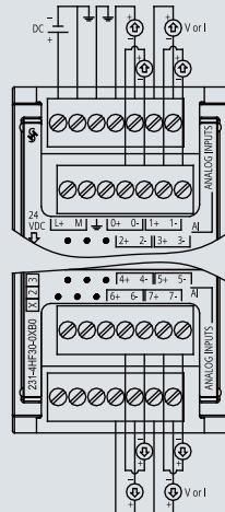
6ES7 231-4HF30-0XB0
