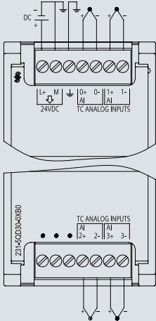
6ES7 231-5QD30-0XB0
