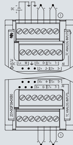
6ES7 231-5QF30-0XB0
