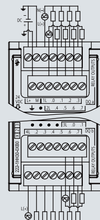
6ES7 222-1HH30-0XB0
