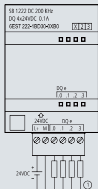
6ES7 222-1BD30-0XB0
