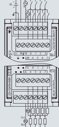
6ES7 223-1QH30-0XB0
