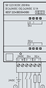
6ES7 223-3BD30-0XB0
