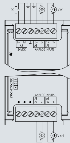
6ES7 231-5ND30-0XB0
