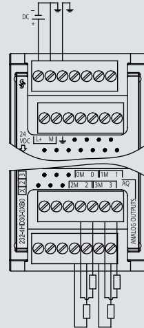
6ES7 232-4HD30-0XB0
