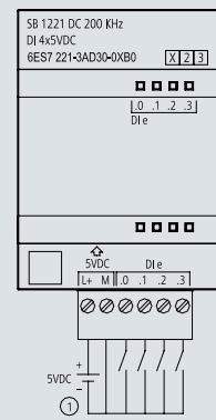
6ES7 221-3AD30-0XB0
