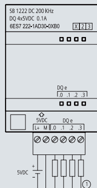
6ES7 222-1AD30-0XB0
