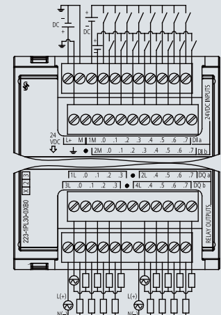
6ES7 223-1PL30-0XB0
