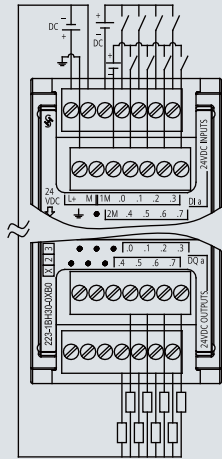
6ES7 223-1BH30-0XB0
