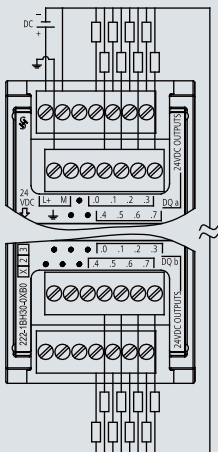
6ES7 222-1BH30-0XB0
