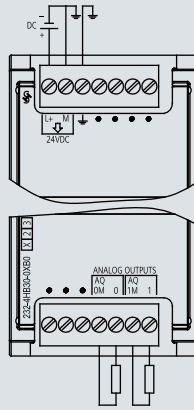
6ES7 232-4HB30-0XB0
