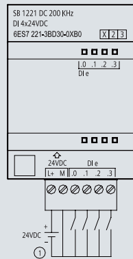
6ES7 221-3BD30-0XB0
