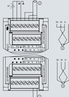
6ES7 231-5PD30-0XB0
