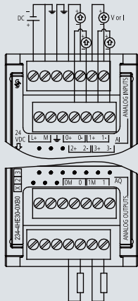
6ES7 234-4HE30-0XB0
