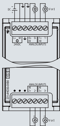
6ES7 231-4HD30-0XB0
