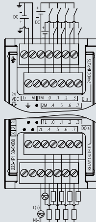
6ES7 223-1PH30-0XB0
